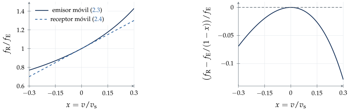
FIGURA 4. Emisor móvil frente a receptor móvil. (Izquierda) f_R/f_E en función de x = v/v_s . (Derecha) Diferencia relativa entre ambas leyes, igual a -x^2/(1-x) y nula para el emisor móvil por construcción. El rango de x se ha ampliado con fines ilustrativos; en el laboratorio |x| \ll 1 .
