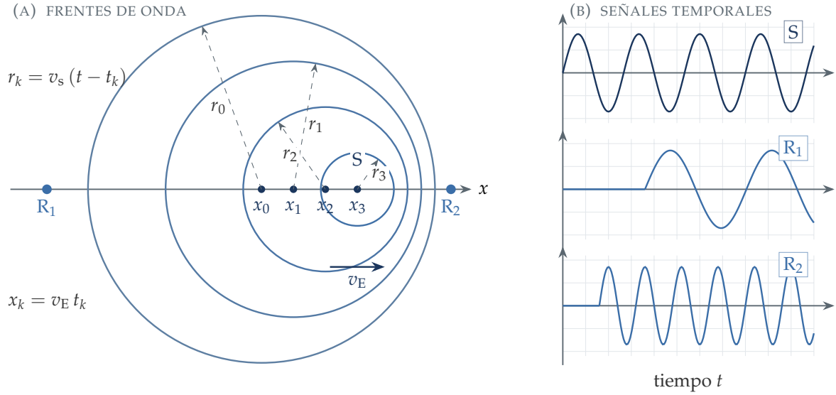
FIGURA 2. Efecto Doppler generado por una fuente S que se desplaza con velocidad v_E . (a) Frenes de onda emitidos en distintos instantes: compresión en el sentido del movimiento y dilatación en el opuesto. (b) Señal emitida frente a las percibidas por los receptores R_1 (menor frecuencia) y R_2 (mayor frecuencia), desfasadas por el tiempo de propagación. Esquema cualitativo, sin escala.
