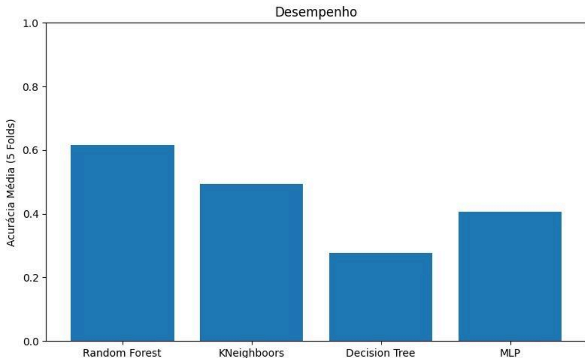
Figura 6: Gráfico representando a acurácia média, utilizando 5 folds no cross-validation, obtida por cada modelo no treinamento com os atributos selecionados por cada modelo pelo algoritmo genético.
