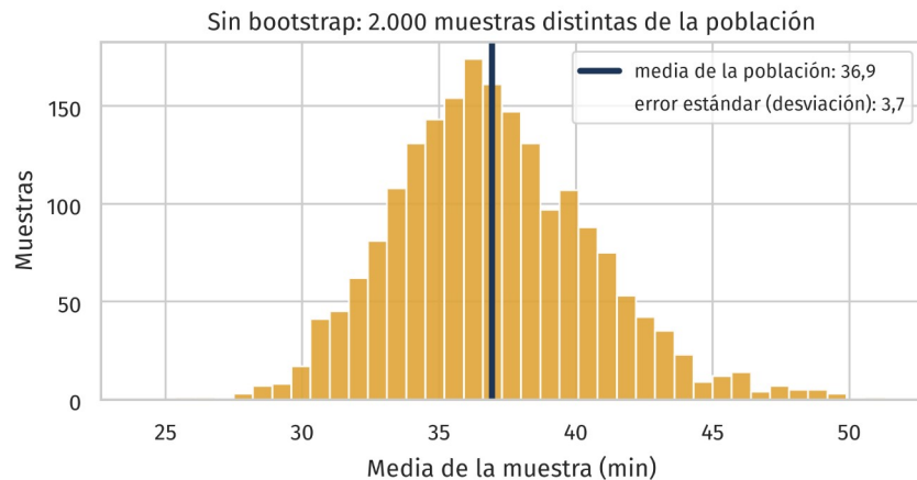
La distribución muestral de la media, por dos caminos
