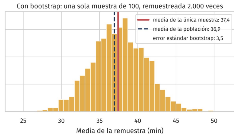
La distribución muestral de la media, por dos caminos
