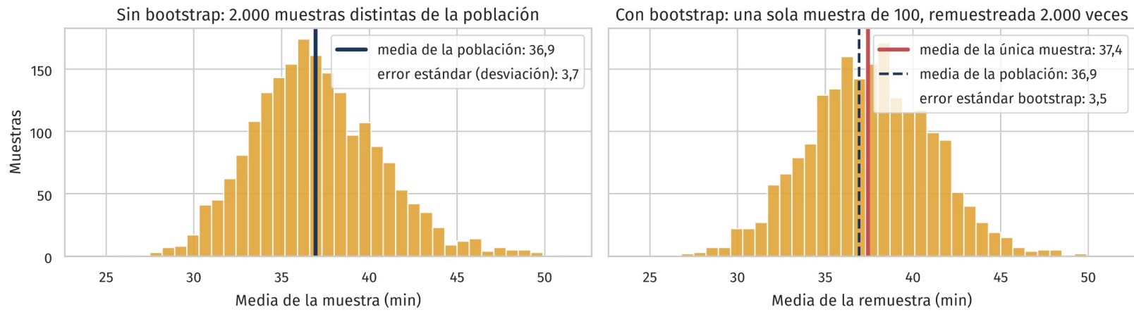
La distribución muestral de la media, por dos caminos
