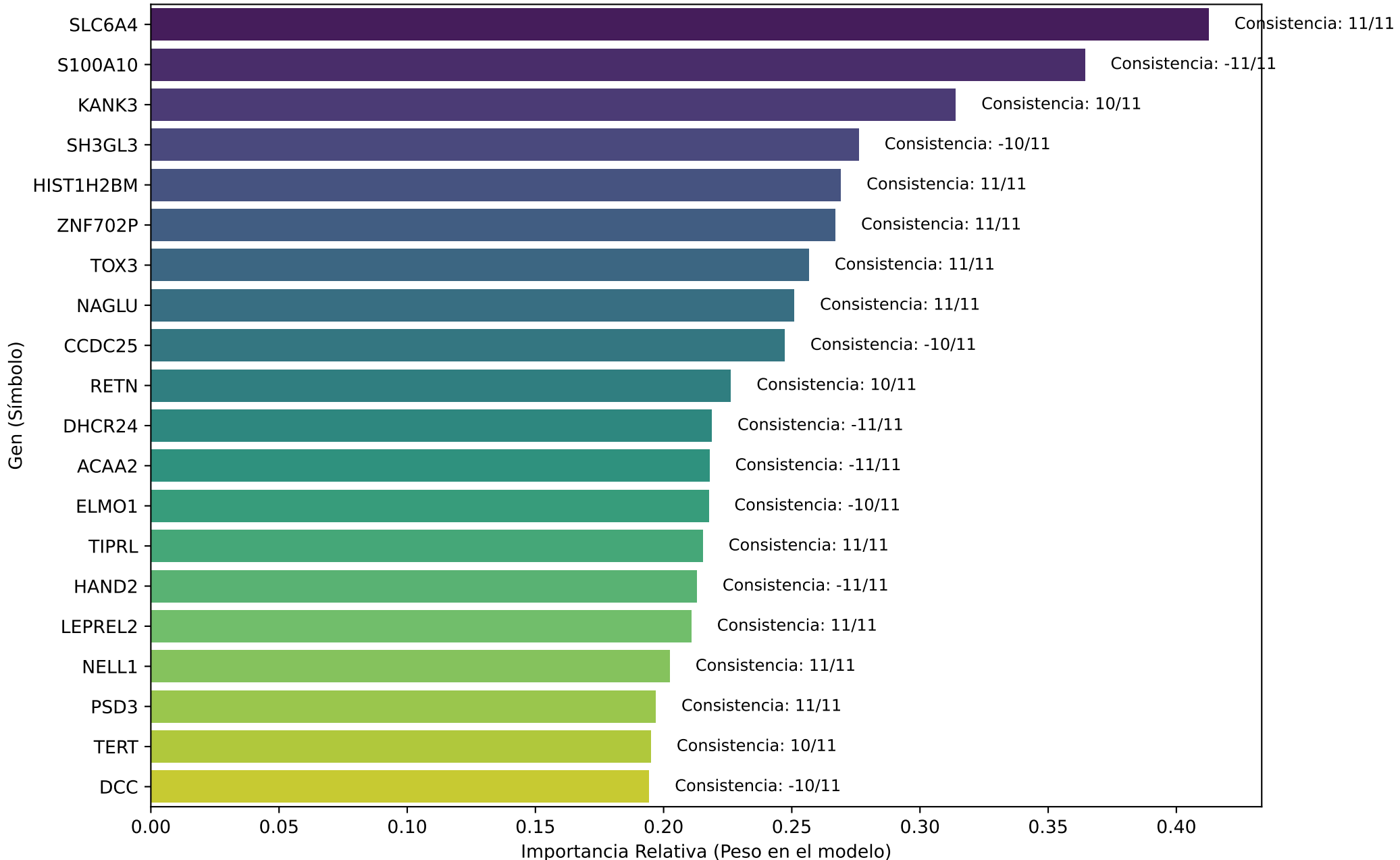
Top 20 Genes por Importancia Media en 11 Estudios
