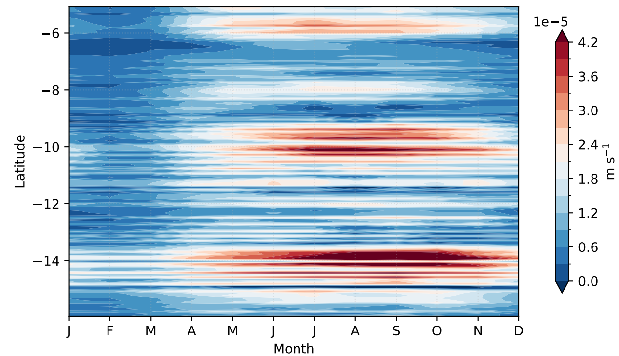
(d) Ek_t
