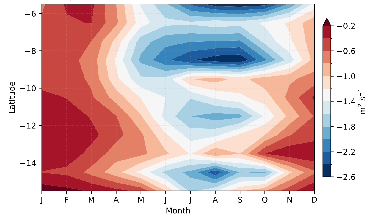
(h) U_{GEO}
