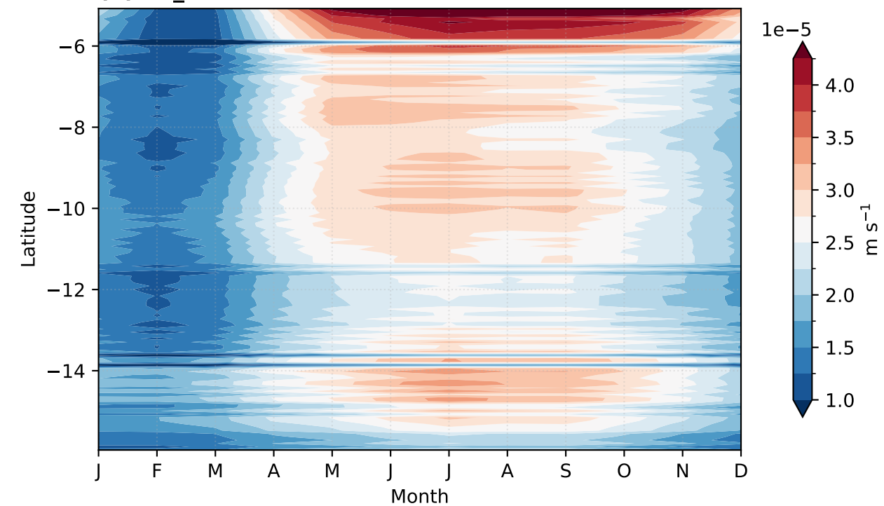
(f) CUI
