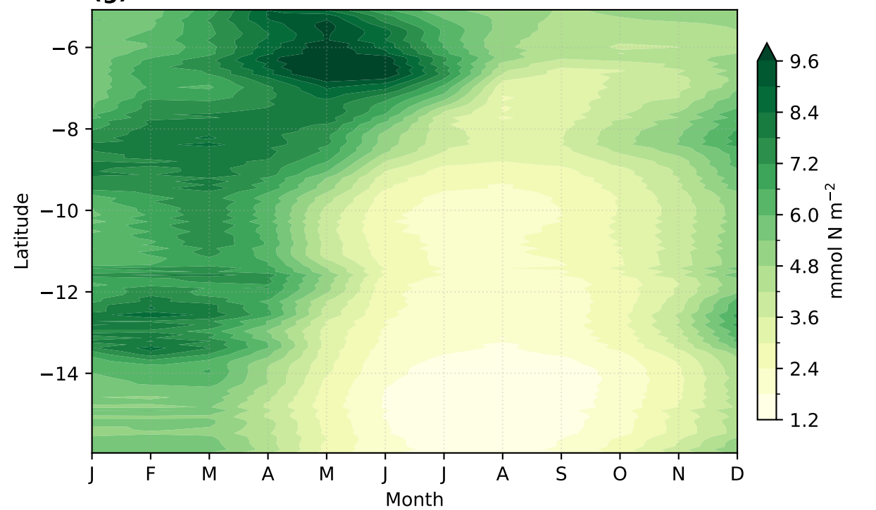
(g) Chl
