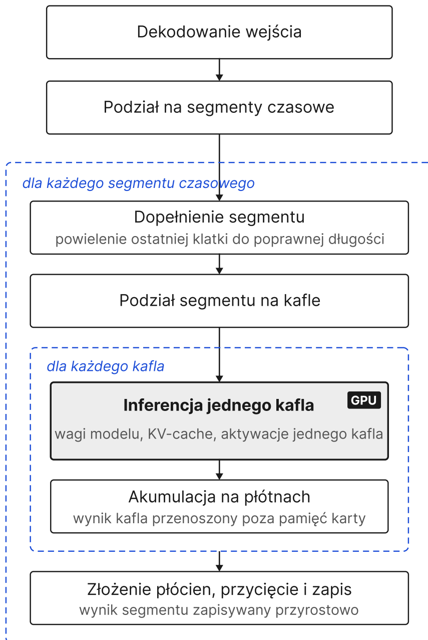
Rysunek 2. Przepływ przetwarzania nagrania w zaimplementowanym potoku
