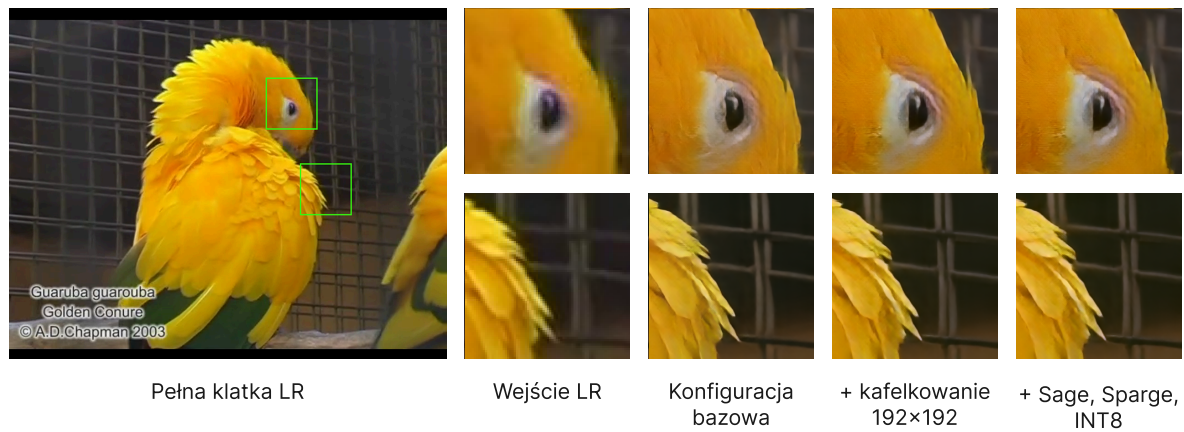
Rysunek 8. Porównanie jakościowe dla zbioru VideoLQ, klip 6, klatka 13. Kolumny: materiał wejściowy, konfiguracja bazowa, konfiguracja bazowa z kafelkowaniem, konfiguracja ze wszystkimi optymalizacjami
