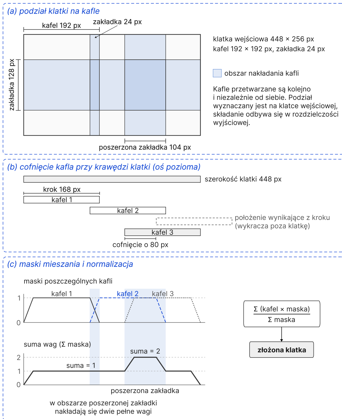
Rysunek 3. Kafelkowanie przestrzenne: (a) podział klatki na kafle z zaznaczonymi obszarami nakładania, (b) cofnięcie kafła wykraczającego poza krawędź klatki, (c) maski mieszania poszczególnych kafli i suma ich wag. Przykład odpowiada wejściu 448 × 256 pikseli, kaflowi 192 piksele i zakładce 24 piksele
