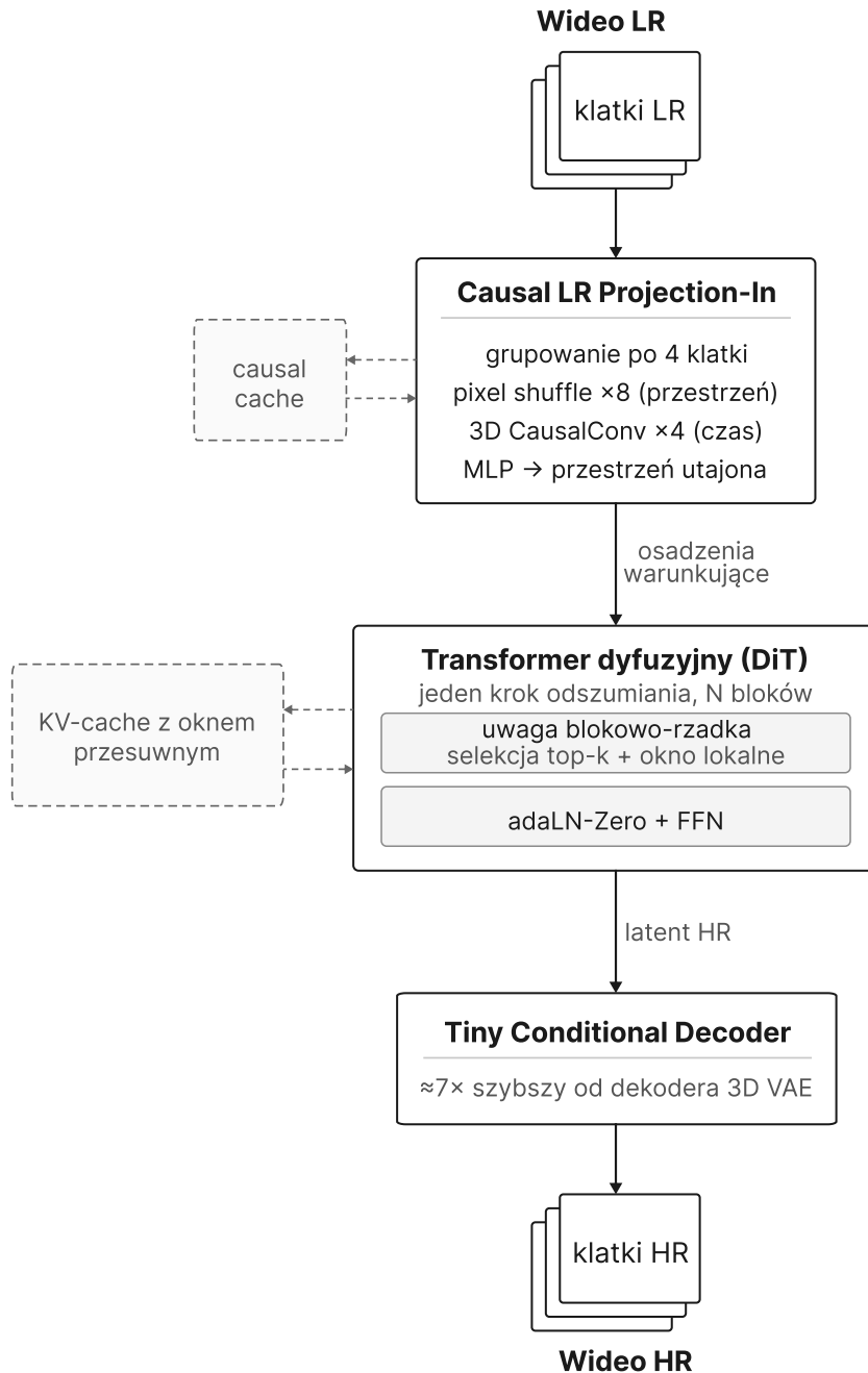
Rysunek 1. Schemat przetwarzania w modelu FlashVSR: projekcja wejściowa, transformer dyfuzyjny z uwagą blokowo-rzadką oraz lekki dekod warunkowy; opracowanie własne na podstawie [1]
