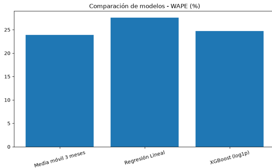
Fig. 34. Comparación de WAPE entre los tres modelos candidatos (holdout final).
