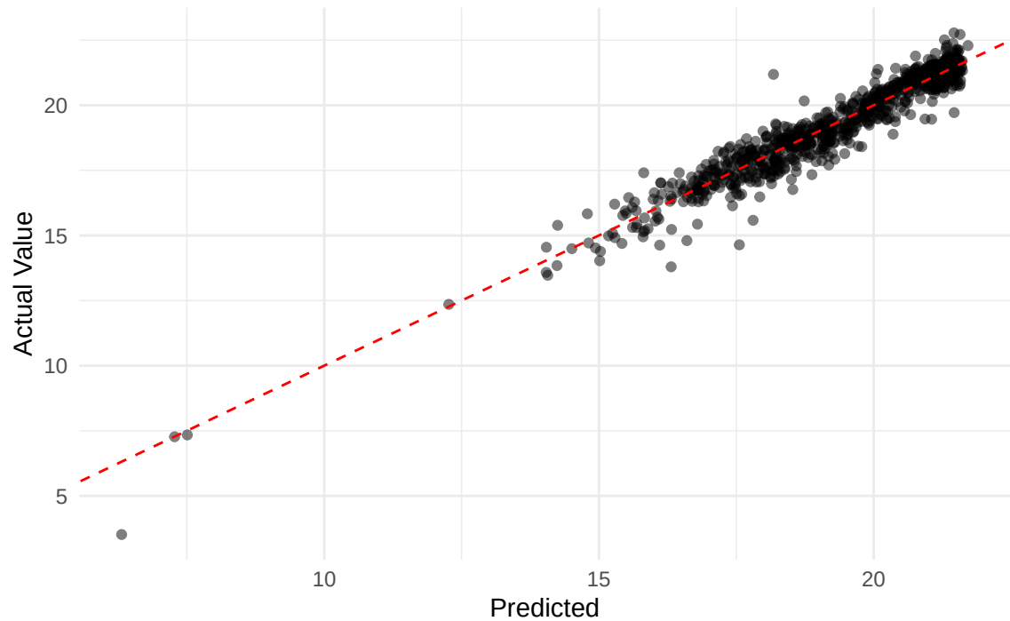
Predicted vs. Actual Values – BMCO
