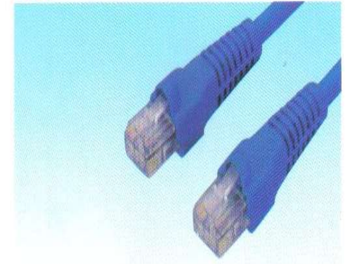
PE 9004 8017: T568B 8078: T568A
