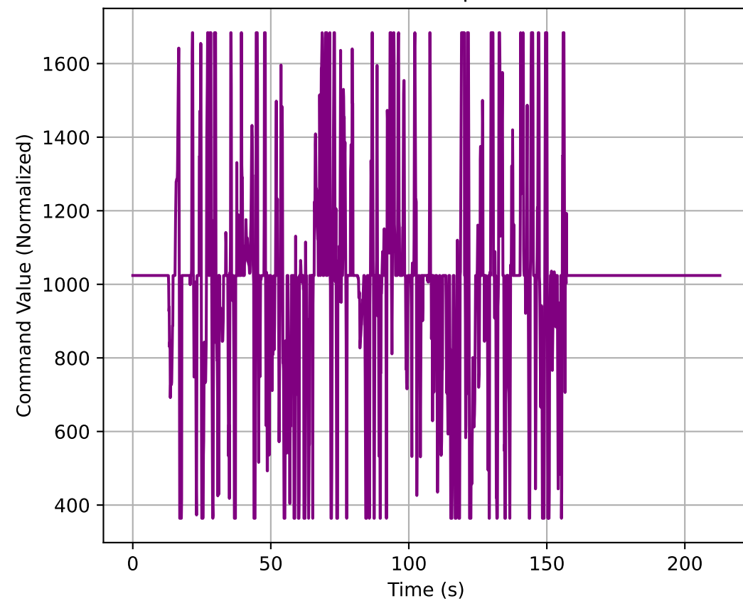
Rudder Input
