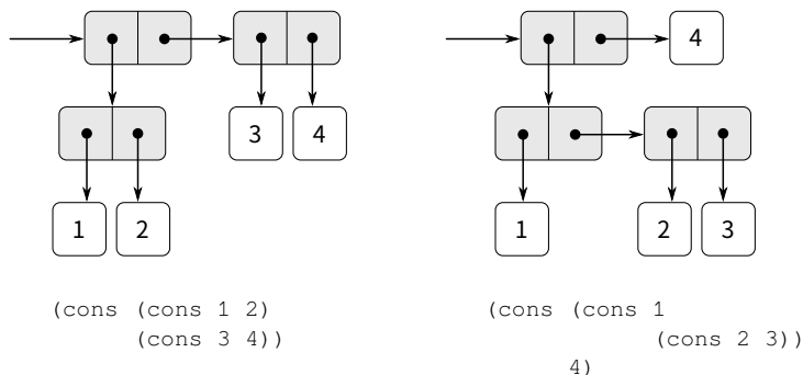
Figure 2.3: Two ways to combine 1, 2, 3, and 4 using pairs. 兩款用對組合 1、2、3 及 4 的方法。
