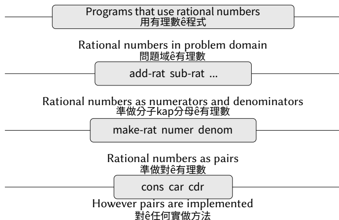
Figure 2.1: Data-abstraction barriers in the rational-number package. 有理數包裹內底層資料抽象化障礙。
