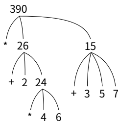
Figure 1.1: Tree representation, showing the value of each sub-combination. 樹 係 表示，展示逐 係 kiáⁿ 組合 係 值。
