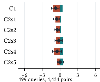
ESCI / GTE / K = 100
