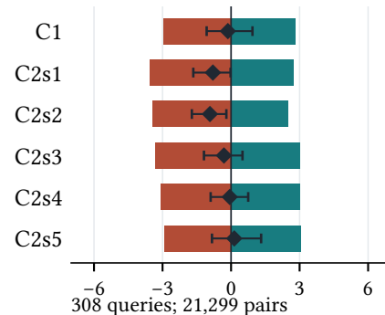
WANDS / GTE / K = 20
