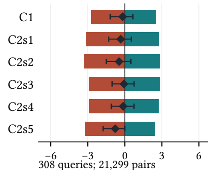
WANDS / GTE / K = 100
