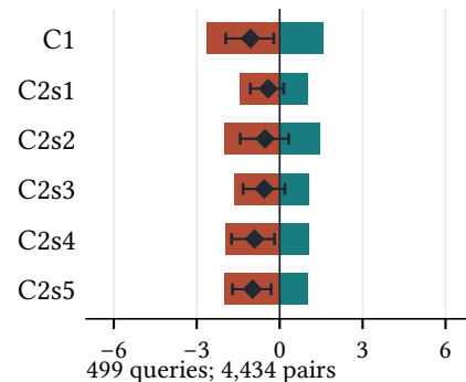
ESCI / GTE / K = 20
