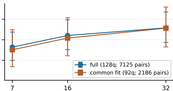
WANDS · BGE · K=100
