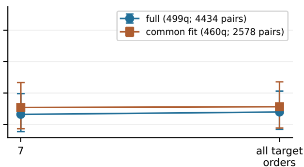
ESCI · BGE · K=100
