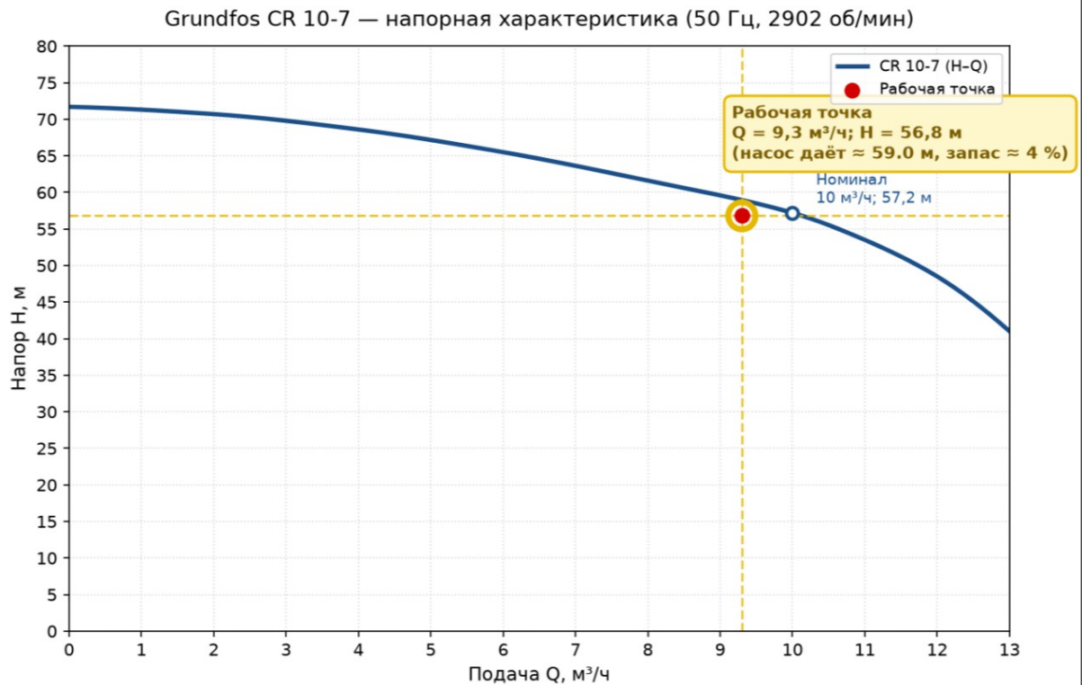
Рисунок 1.1 – Напорная характеристика насоса Grundfos CR 10-7 (построена по паспортным точкам: H = 71,7 \text{ м} при Q = 0 ; H = 57,2 \text{ м} при Q = 10 \text{ м}^3/\text{ч} ) и рабочая точка установки
