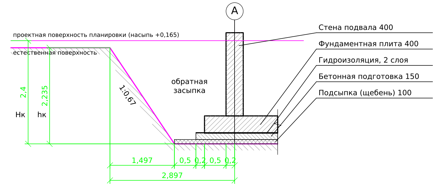
1-1 (фрагмент) М 1:50
