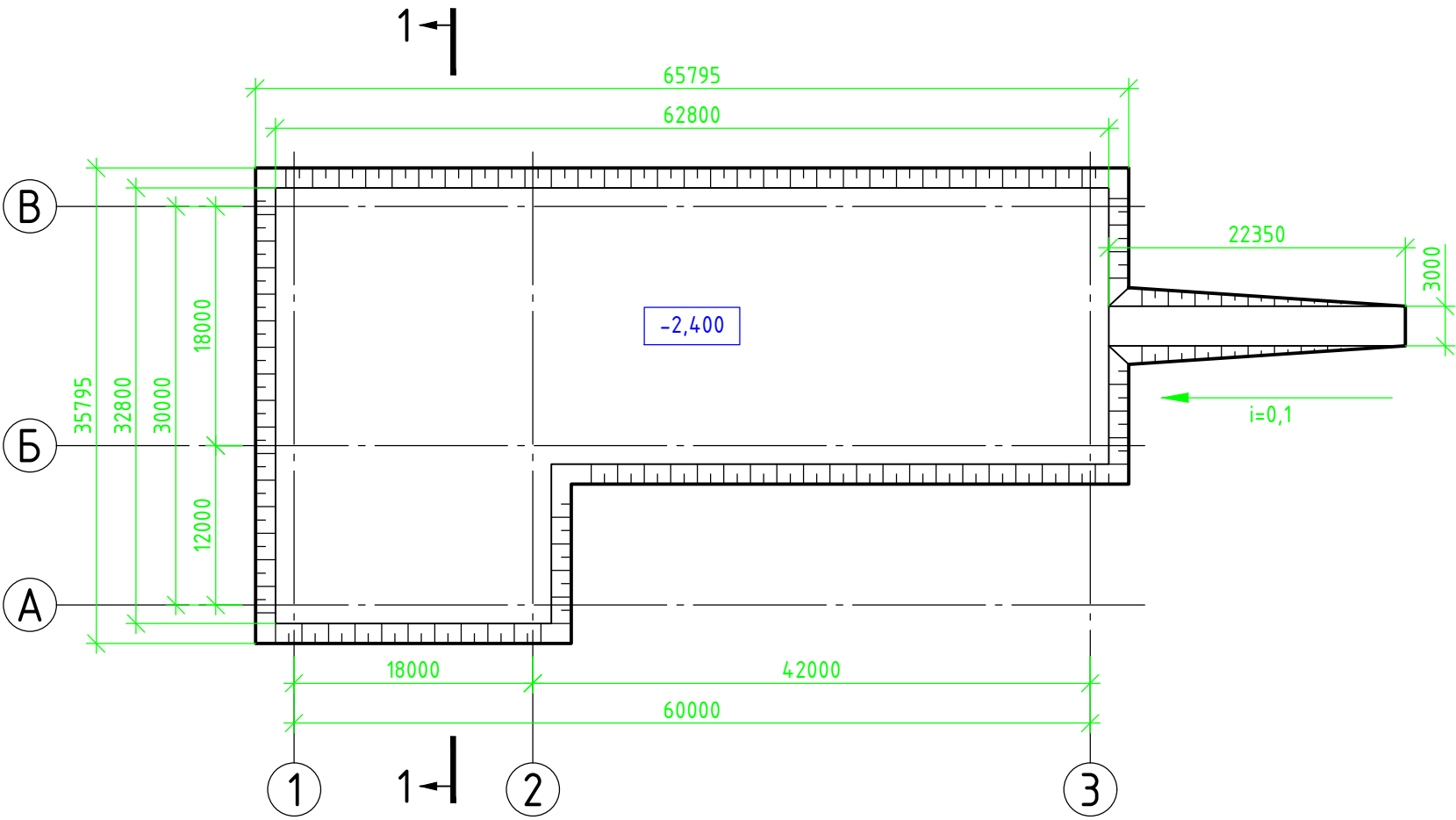
План котлована М 1:500
