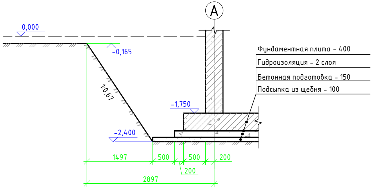
Разрез 1-1 М 1:50
