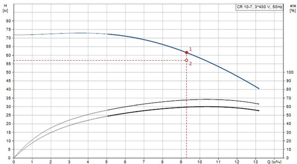
Рисунок 1.1 – Характеристика насоса Grundfos CR 10-7, 3 \times 400 \text{ В} , 50 Гц [13]: 1 – рабочая точка; 2 – требуемый напор установки
