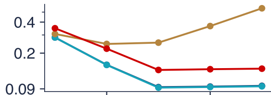
DGP: AR(3)
