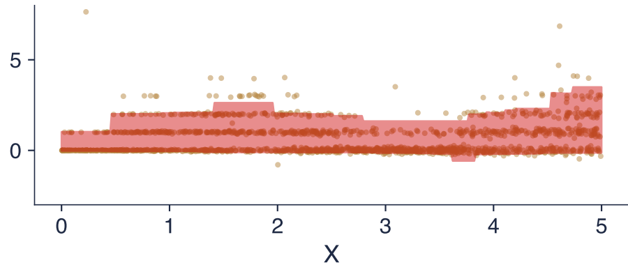
CQR (quantile models)
