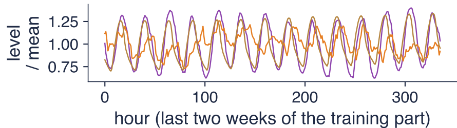
— M4 H1 — M4 H101 — M4 H301
