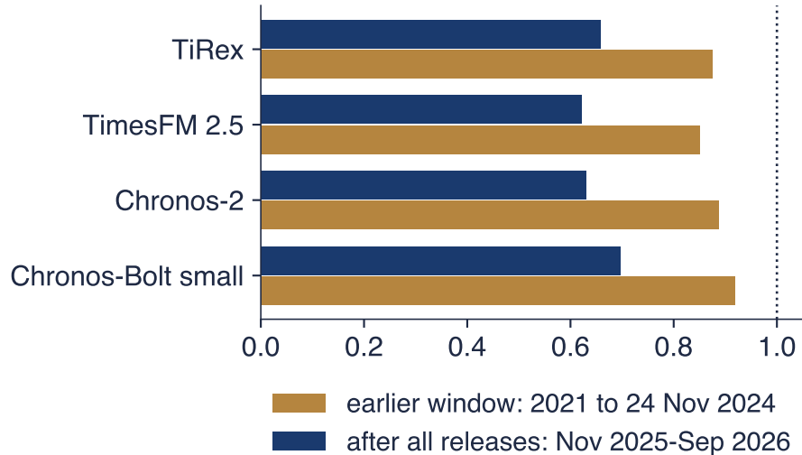
Bitcoin RV: QLIKE / HAR
