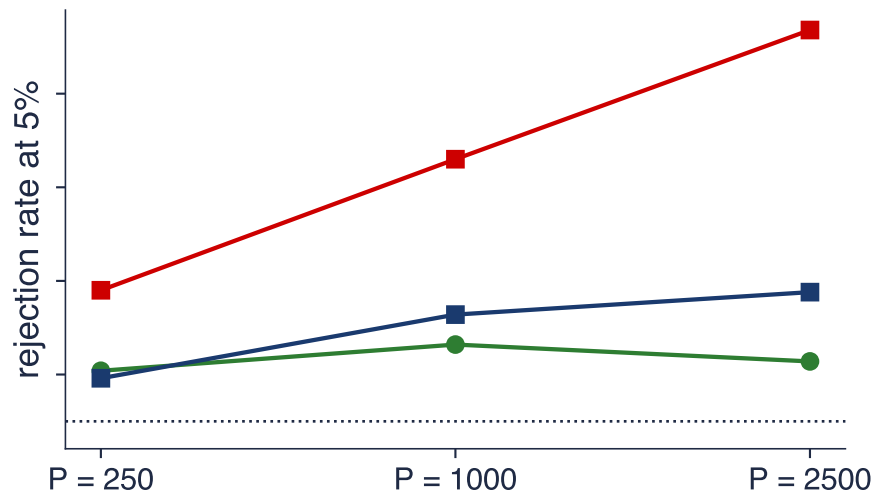
DQ test, VaR 1%
