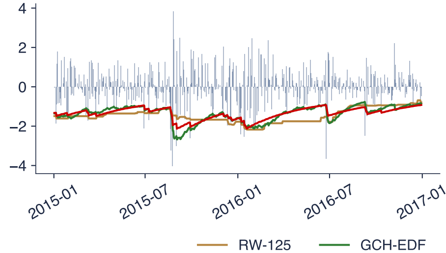
VaR 5% (return quantile)
