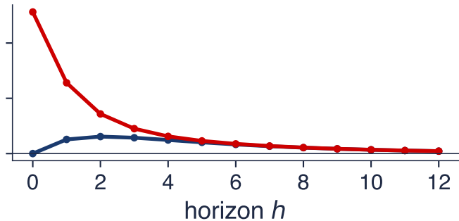
shock \varepsilon_2
