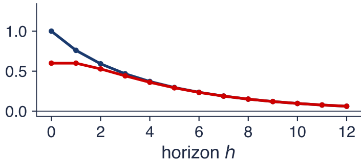
shock \varepsilon_1
