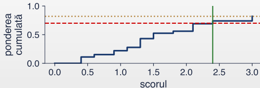
— ponderea cumulată - - - 1 - \alpha = 0,7 ..... 1 - \tilde{w}_{n+1} — \hat{q} ponderat
