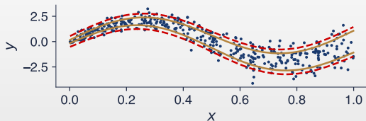
• puncte de test — cuantile brute 10%, 90% - - - banda CQR, \pm \hat{q}
