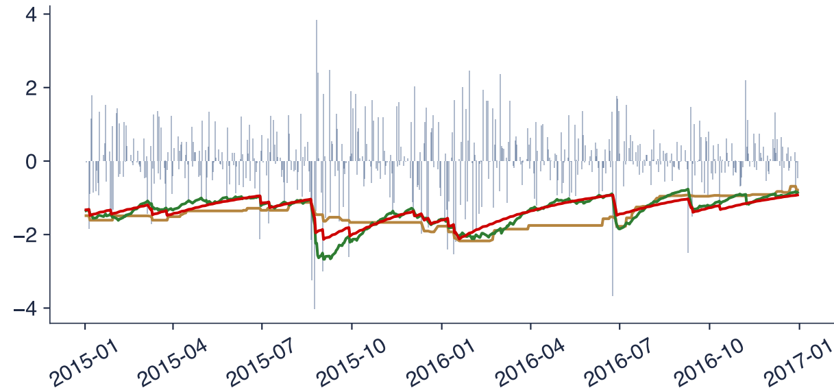
VaR 5% (return quantile)
