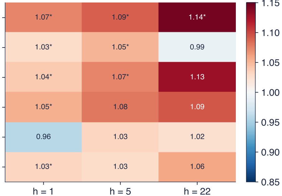
HGB / HAR (QLIKE)
