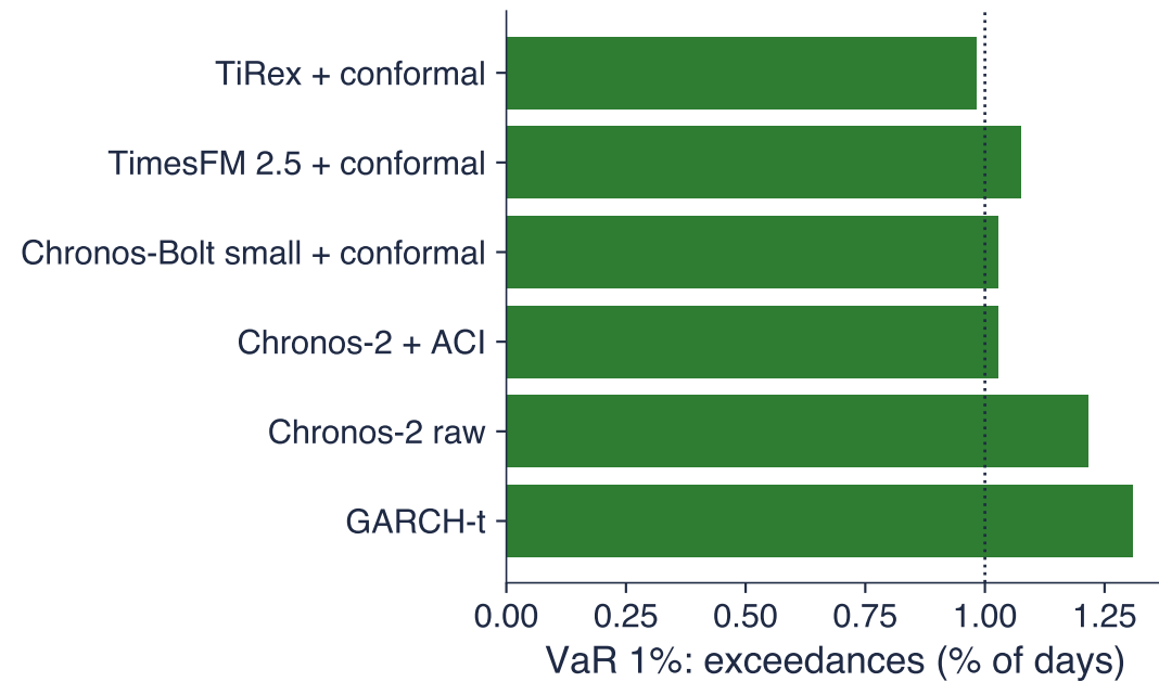
BET
