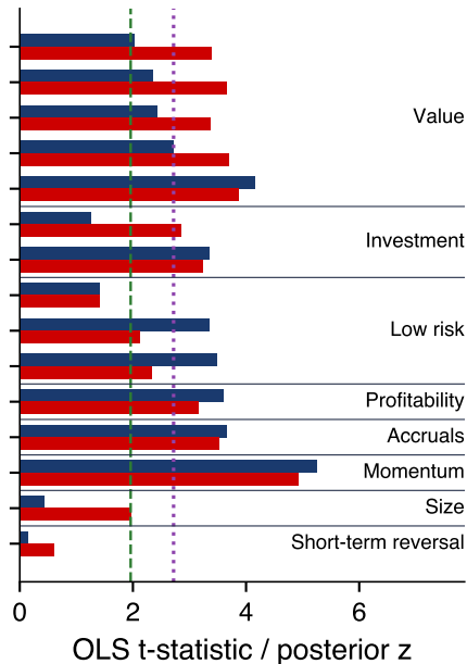
OLS t versus posterior z
