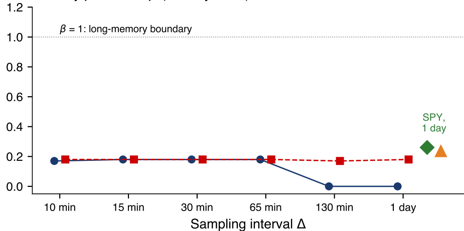
Memory parameter \hat{\beta} (Cauchy class)
