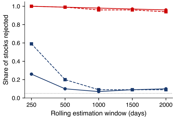
GARCH(1,1)
