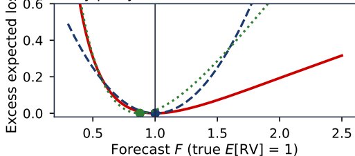
Noisy proxy: minimisers
