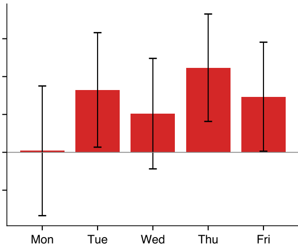
BET (Romania): equal-means p = 0.31
