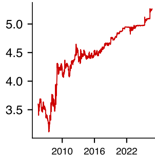
EUR/RON (BNR)
