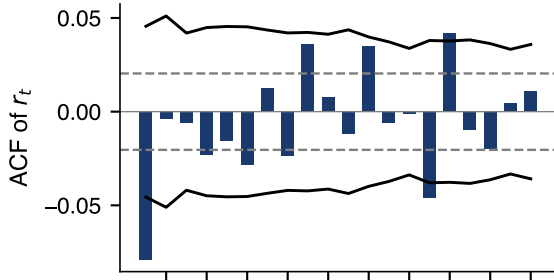
EUR/RON (T = 5,352)
