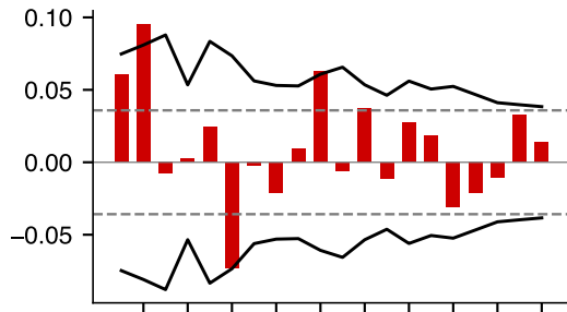
Bitcoin (T = 4,384)
