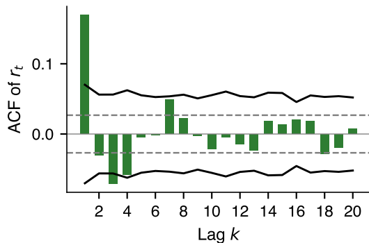
EUR/RON (T = 5,352)
