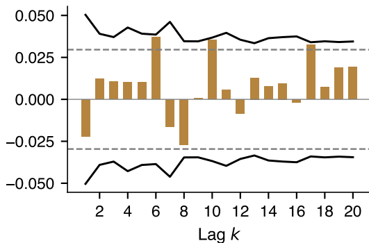
Bitcoin (T = 4,384)
