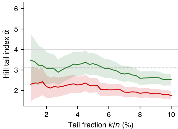
BET-TR (Romania)
