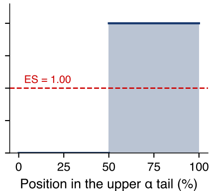
F1: P(L=2) = \alpha/2 , P(L=0) = 1 - \alpha/2
