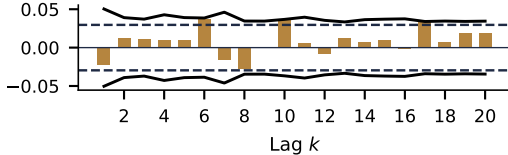
Bitcoin (T = 4,384)
