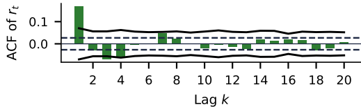
EUR/RON (T = 5,352)
