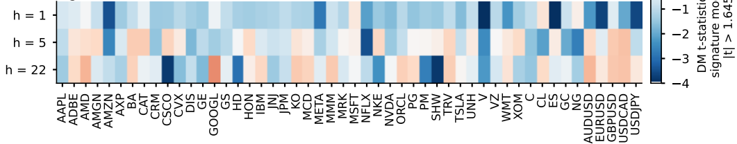
Sig-LK vs HAR (DM t-statistic, QLIKE)
