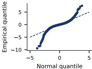
Quantile-quantile plot
