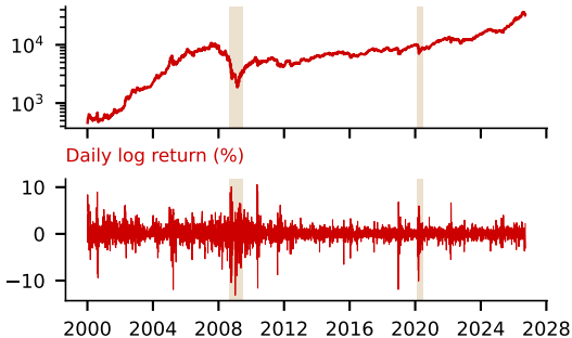
BET (Romania): close (log scale)
