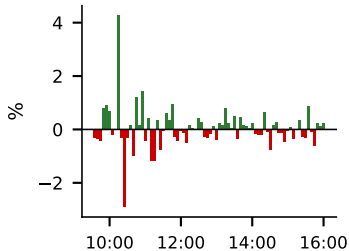
78 returns
