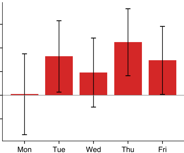
BET (Romania): equal-means p = 0.29
