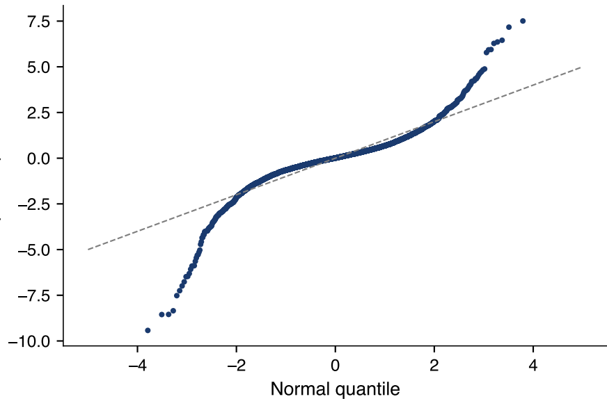
Quantile-quantile plot
