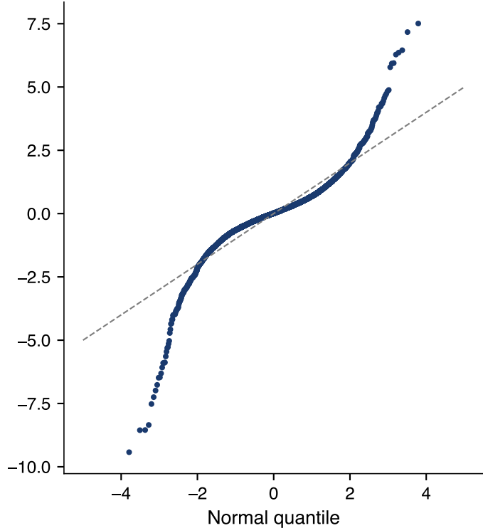
Quantile-quantile plot
