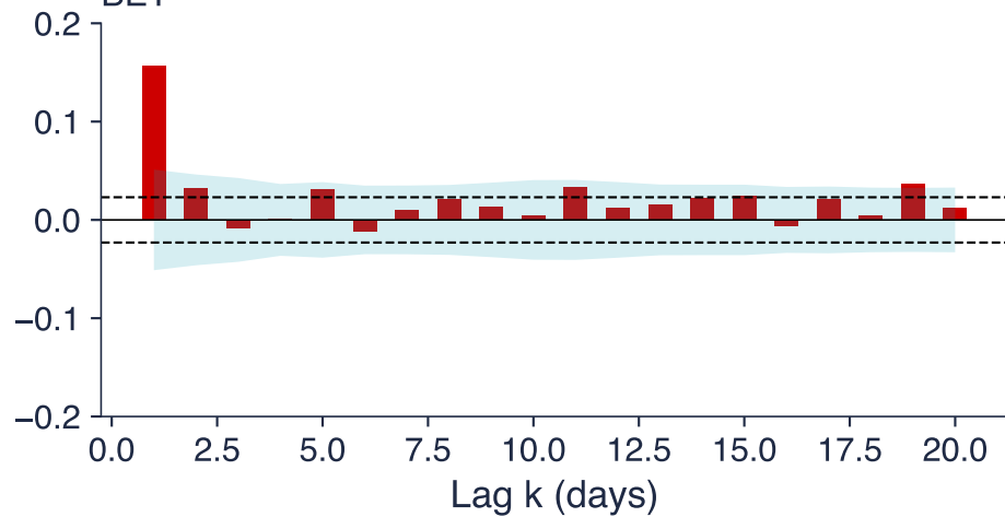
BET
