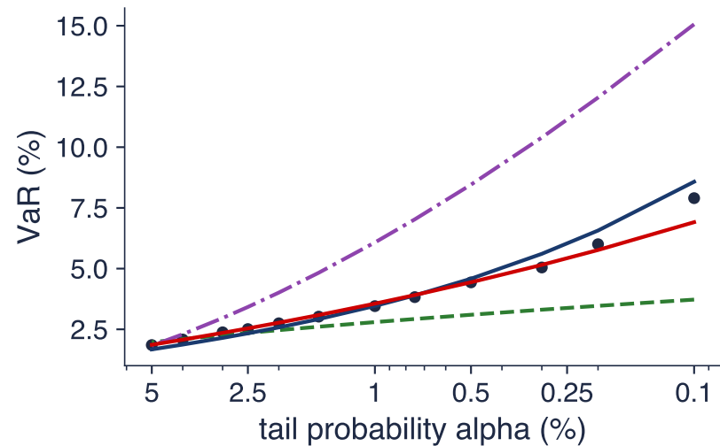
S&amp;P 500
